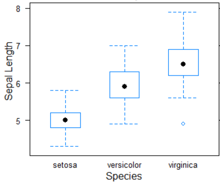
Iris Boxplot
