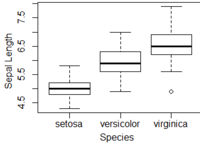
Iris Boxplot
