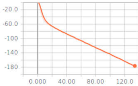
da_loss_real
