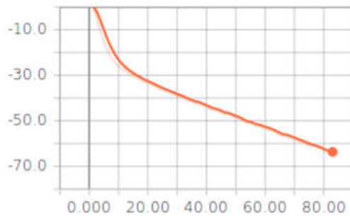
da_loss
